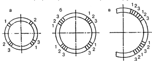
Рис. 3. Схема вырезки образцов для механических испытаний
